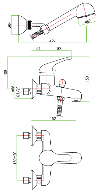
FIG. DESCRIZIONE MATERIALE PESO (gr) Miscelatore vasca con duplex 2180
